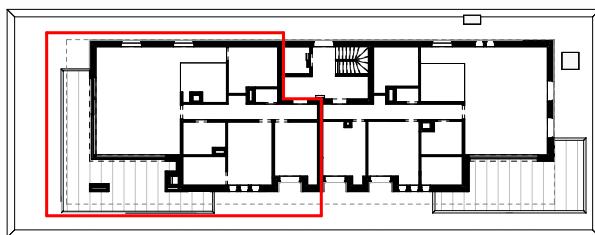
Verdieping +2
